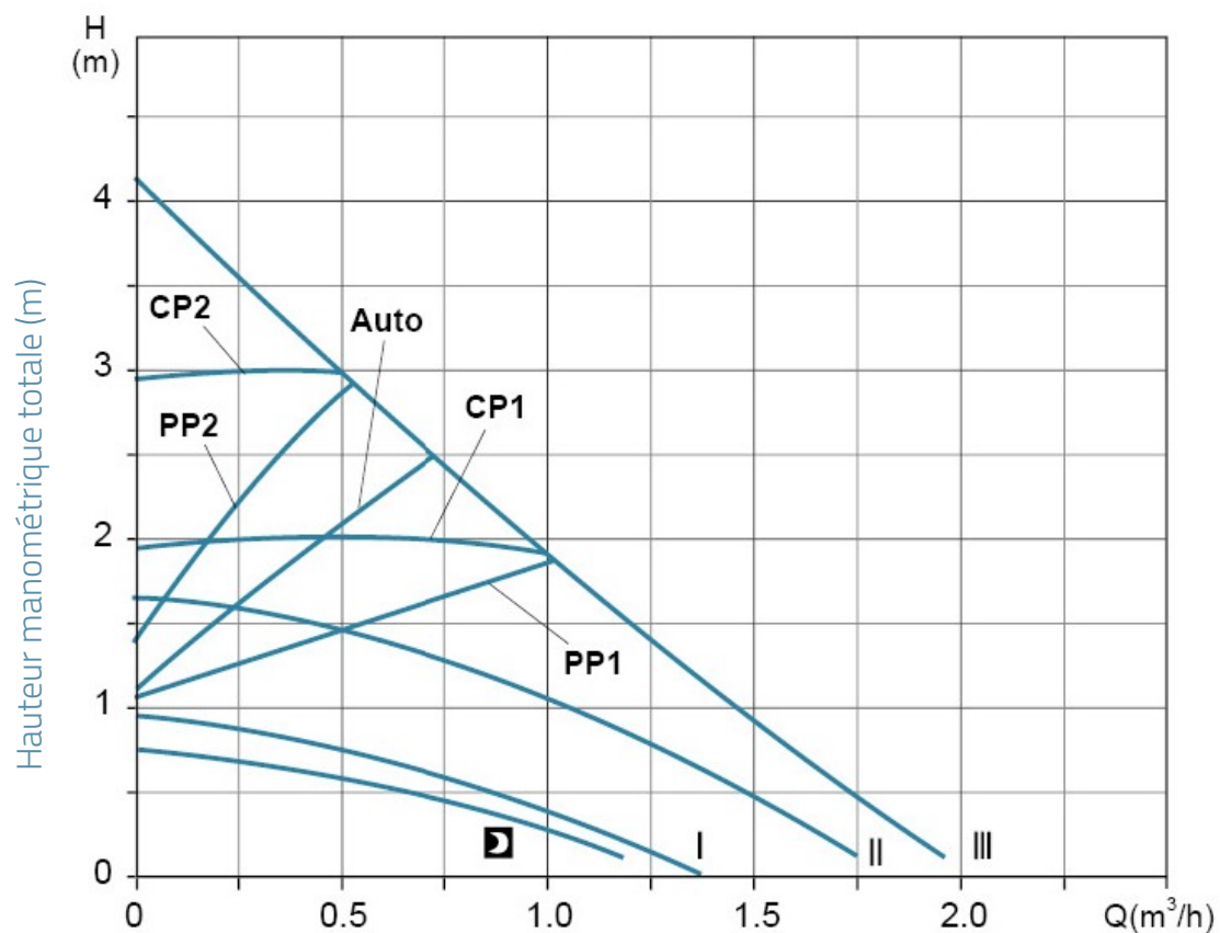
ARPXX-40 Q-H
