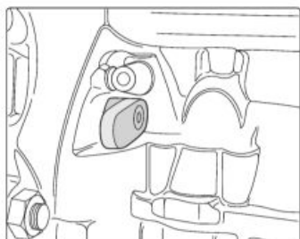
Timing locking set for engines 1.2 6V / 12V (chain) Zestaw blokad rozrządu silników 1.2 6V / 12V (łańcuch)
